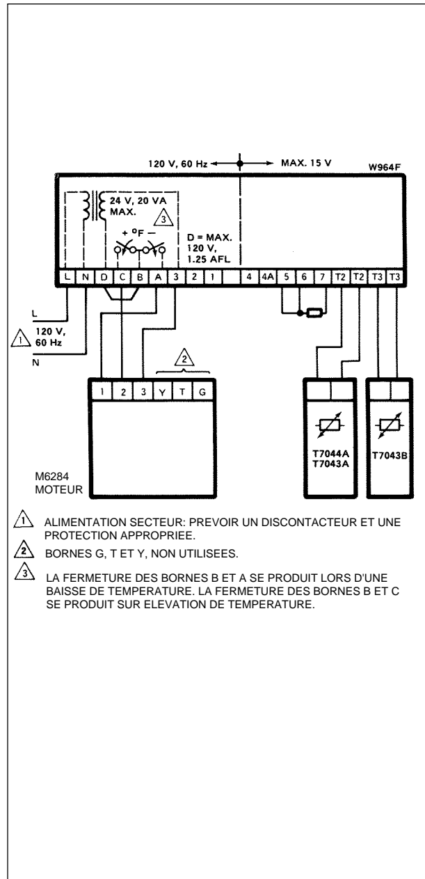
Figure 11 - Câblage pour un contrôleur W964F et servomoteur sans transformateur interne
