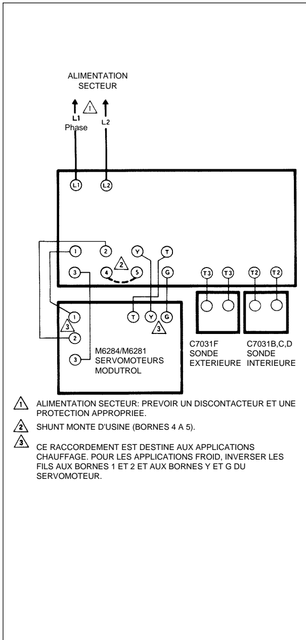
Figure 10 - Versions d'usine sans transformateur interne utilisées avec un contrôleur extérieur W902 en application chaud ou froid.
