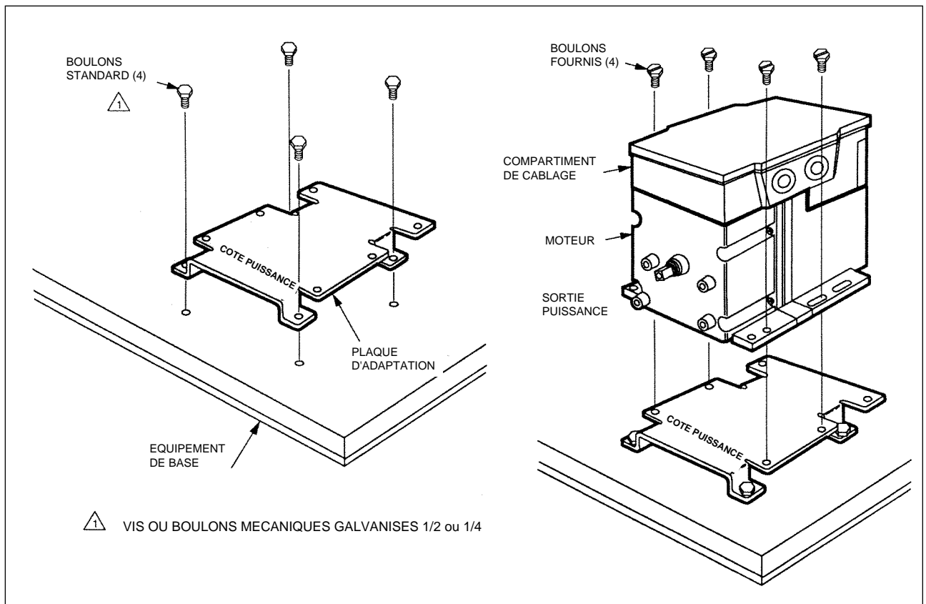
Figure 3 - Montage du moteur avec plaque. Avec cette option, la plaque d'adaptation est préalablement montée sur l'équipement avec les boulons standard. Le servomoteur est ensuite monté sur la plaque en utilisant les boulons fournis qui sont vissés dans les trous filetés de la plaque.
